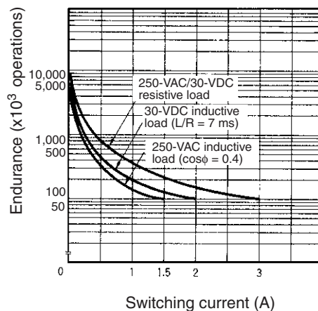
G2RK-2A, G2RK-2
