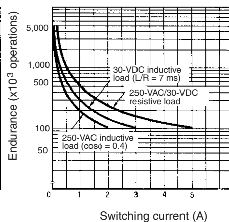
G2R-1Z4, G2R-1AZ4
