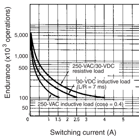
G2R-24, G2R-2A4
